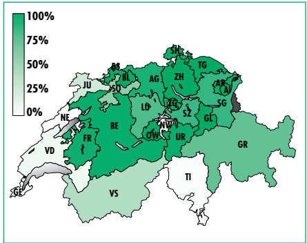
Pourcentage des communes ayant introduit la taxe au sac dans les cantons suisses (chiffres 2000). 60 % des communes ont adopté ce système, soit 67% de la population.
